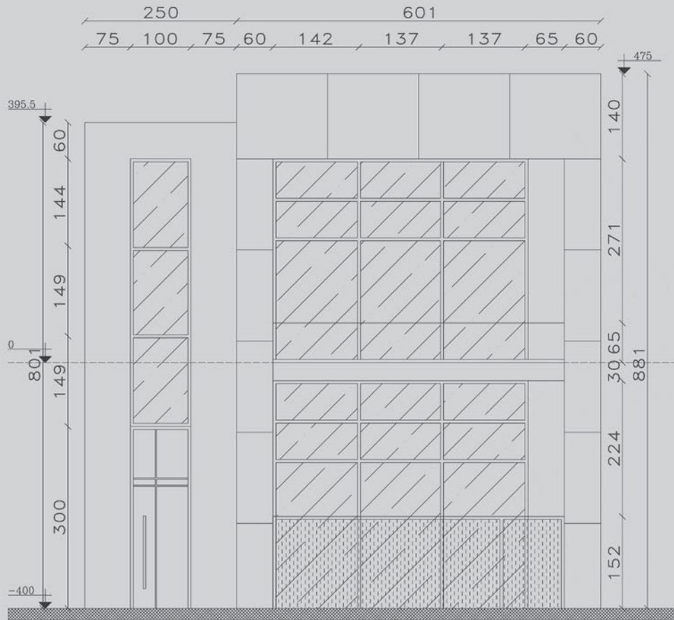
الواجهة الأمامية FRONT FACADE
