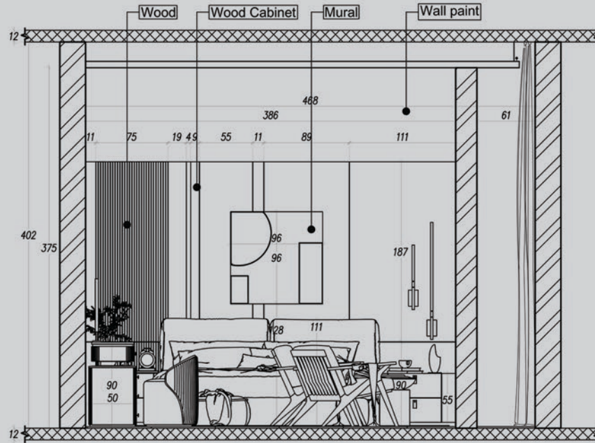
غرفة النوم الرئيسية PRIMARY BEDROOM
